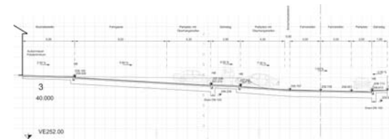
Querprofil Stegersbach Kastellstr.
