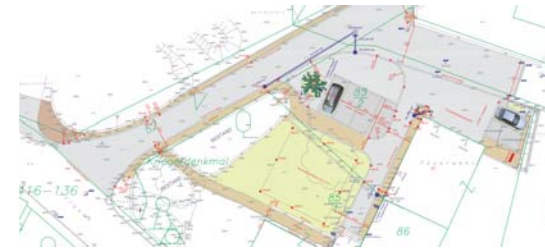
Lageplan Kreisegg
